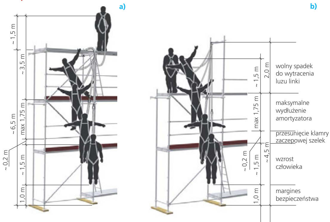
Rys. 2. Zależność bezpiecznej wysokości upadku od umiejscowienia punktu konstrukcji stałej: a) montaż pierwszej ramy; b) montaż kolejnych pól rusztowania.
