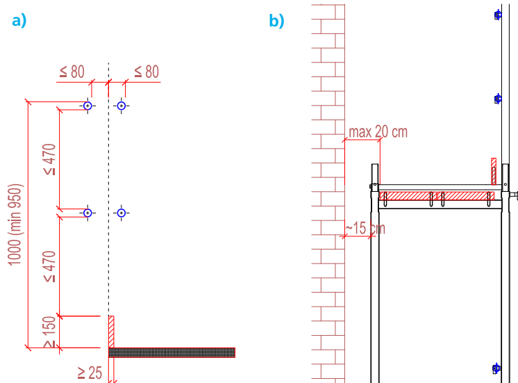
Rys. 12. Balustrada na rusztowaniu:
